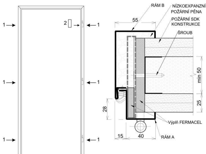
1 - montážní kotva 2 - identifikační štítek s požární odolností uzávěru od výrobce dveří
